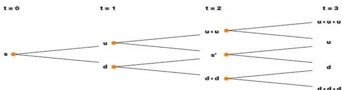
Рис. 2. «Дерево решений» трехступенчатой биномиальной модели
